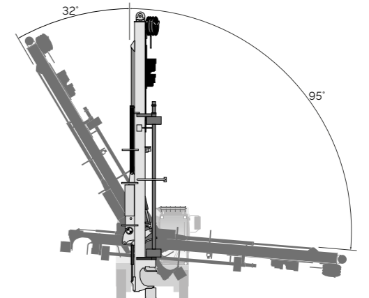
推进梁摆动角度 - 标准推进梁
