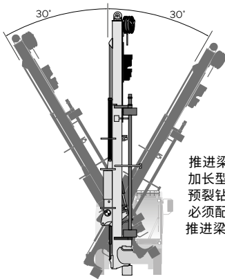
推进梁摆动角度 - 标准推进梁
