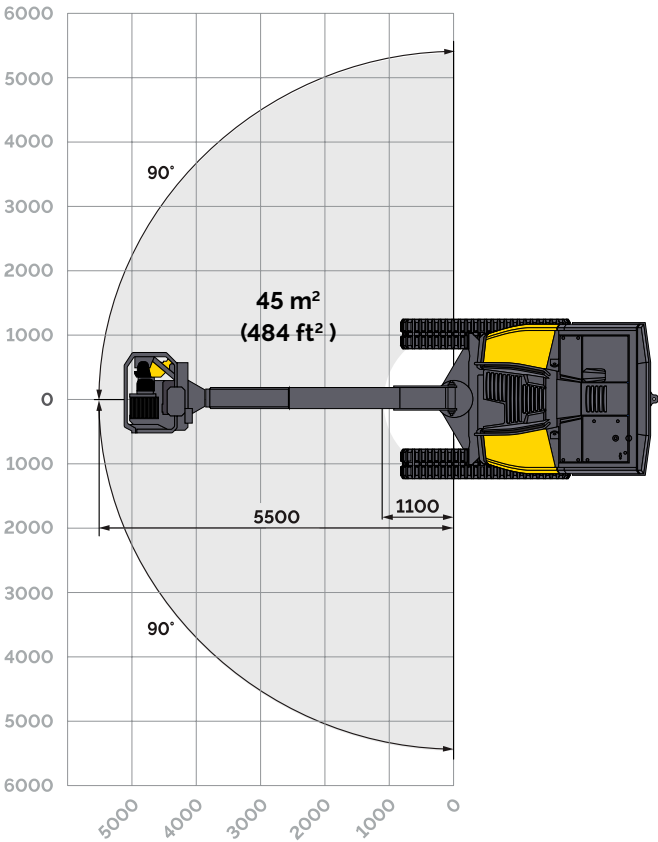
Område för horisontell borrar (mm) – 90/90
