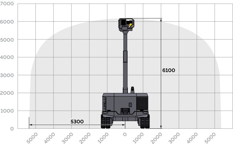
Vertikal täckarea (mm) – 90/90
