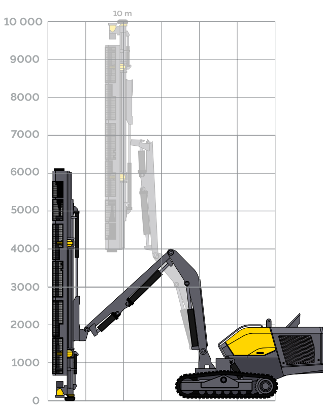
Vertikal räckvidd uppåt
